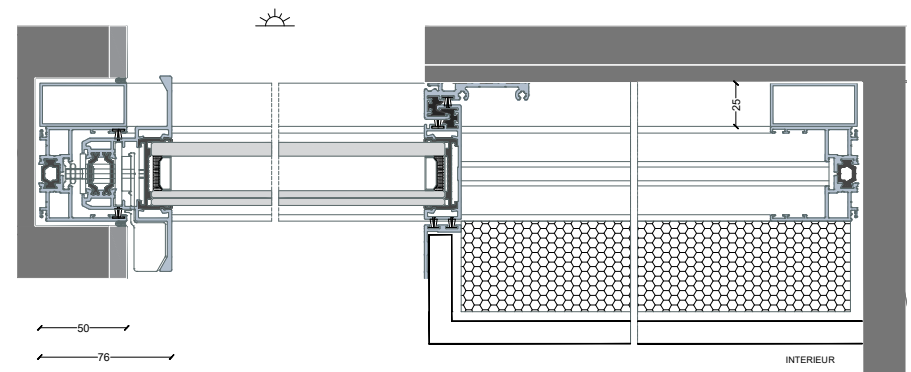
Détail par défaut
