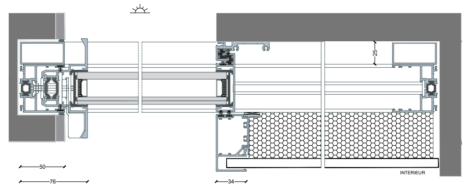
Détail variante chicane galandage
