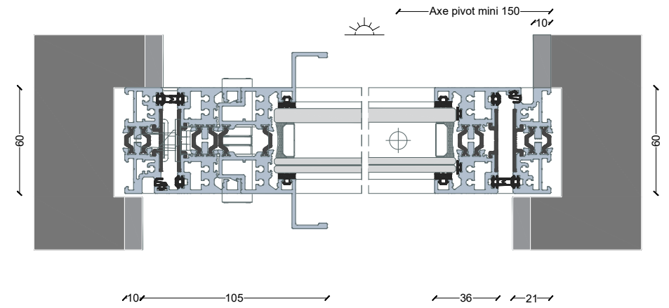
Version porte pivot sur monorail 1 vantail
